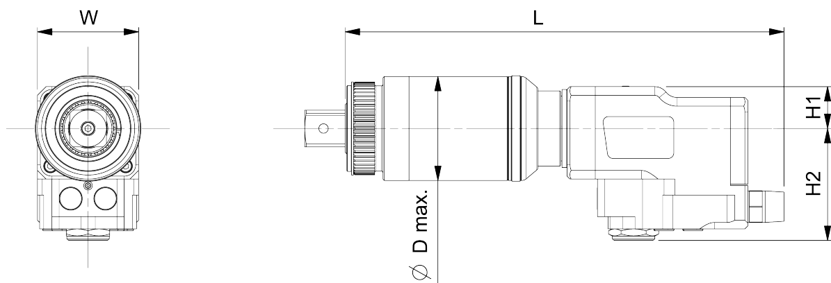
FIGUR 13 – Dimensjoner
